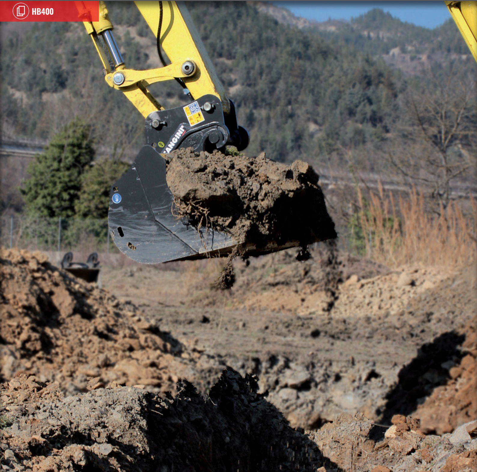
BÖSCHUNGSLÖFFEL MIT VORGEZOGENEM PROFIL FÜR LEHMIGE UND FEUCHTE BÖDEN. ZUM EINEBNEN UND RÄUMEN VON STRASSEN, GRÄBEN UND BÖSCHUNGEN. SCHNEIDE AUS 400HB-STAHL.
