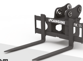
FORCA PALLET FK PER ESCAVATORE
