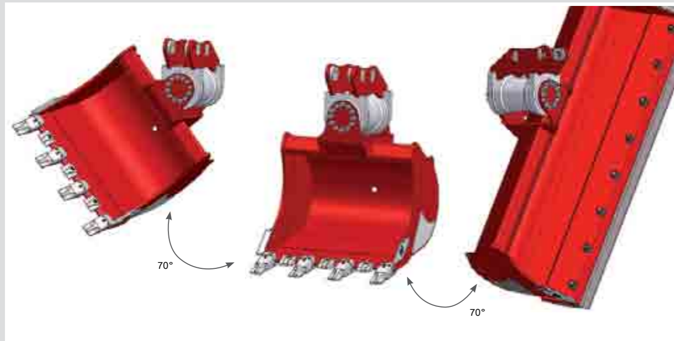
APPLICAZIONE SU BENNE E GRADI DI INCLINAZIONE
